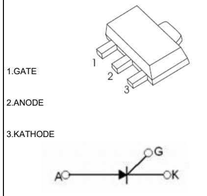
SOT-89-3L
